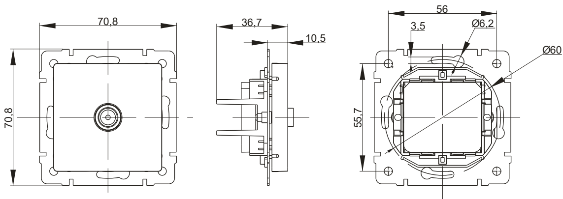
Телевизионная розетка
