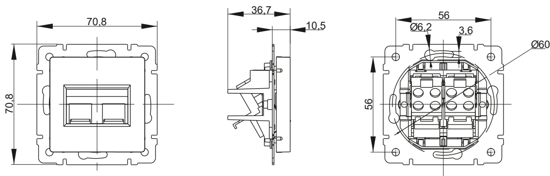
Двойная (компьютерная+телефонная) розетка
