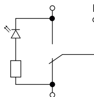
Выключатель одноклавишный проходной с индикацией
