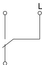
Выключатель одноклавишный проходной
