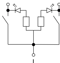
Выключатель двухклавишный с индикацией
